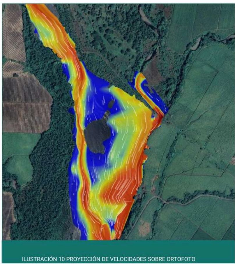
ILUSTRACIÓN 10 PROYECCIÓN DE VELOCIDADES SOBRE ORTOFOTO
