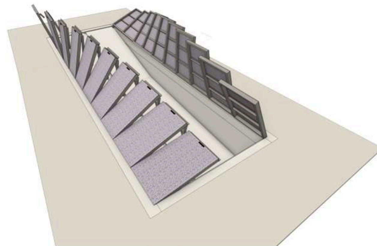
VISTA 2 APERTURA DE COMPUERTAS / PISCINA
